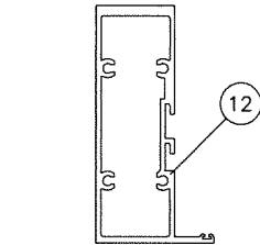
JAMB 'J5' (LEVEL 'D' & 'E' IMPACT)
